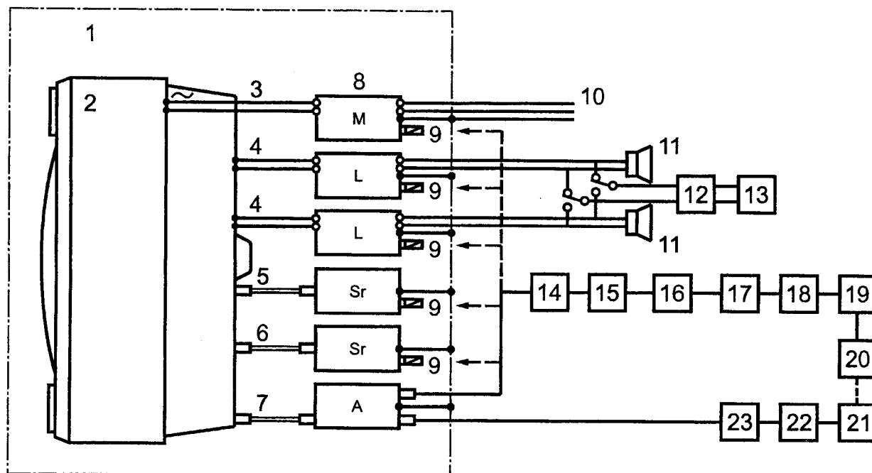
1 — пластина заземления; 2 — испытуемый телевизор; 3 — провод электропитания; 4 — провод подключения громкоговорителя; 5 — кабель блока дистанционного управления; 6 — кабель для передачи звуковых сигналов; 7 — антенный кабель; 8 — устройства связи; 9 — резистор сопротивлением 50 Ом; 10 — к сети электропитания; 11 — громкоговоритель; 12 — полосовой фильтр; 13 — вольтметр переменного тока; 14 — аттенюатор; 15 — фильтр нижних частот; 16 — усилитель мощности (при необходимости); 17 — аттенюатор; 18 — переключатель; 19 — генератор испытательных сигналов; 20 — генератор звуковых частот; 21 — генератор телевизионных испытательных сигналов; 22 — каналный фильтр; 23 — аттенюатор
