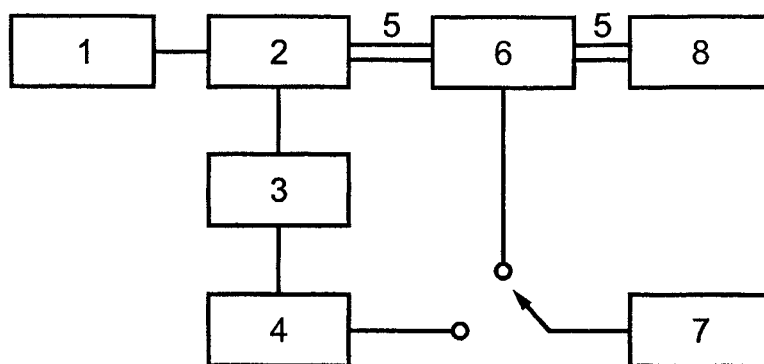
1 — генератор телевизионных испытательных сигналов; 2 — высокочастотный смеситель; 3 — согласующий аттенюатор; 4 — регулируемый аттенюатор; 5 — измерительный кабель; 6 — поглощающие клещи; 7 — генератор испытательных сигналов; 8 — испытуемый телевизор
