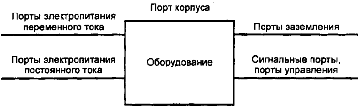
Рисунок 1 — Примеры портов
