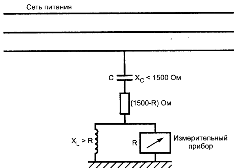
Рисунок 4 — Схема измерения напряжения ИРП на сетевых зажимах по 6.2.3
