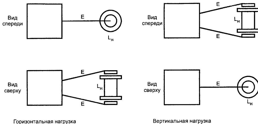
Рисунок 3 — Взаимное расположение медицинского оборудования (конденсаторного типа) и эквивалента нагрузки (см. 6.5.1.1)
