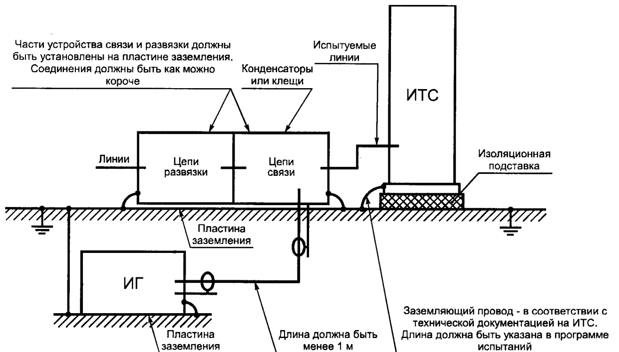
Рисунок 6 — Схема испытаний на устойчивость к НИП
