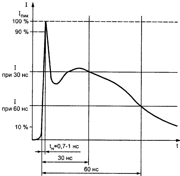
Рисунок 2 — Типовая форма импульса разрядного тока на выходе ИГ
