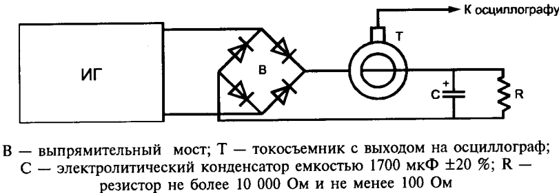
Рисунок В.1 — Схема измерения нагрузочной способности ИГ по пиковому току
