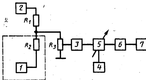
Структурная схема измерения внеполосных излучений радиопередатчиков морской подвижной службы
