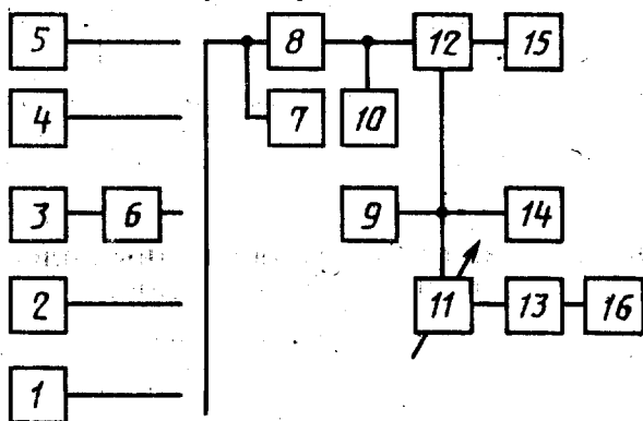
Структурная схема измерений ширины полосы радиочастот и внеполосных излучений радиопередатчиков
