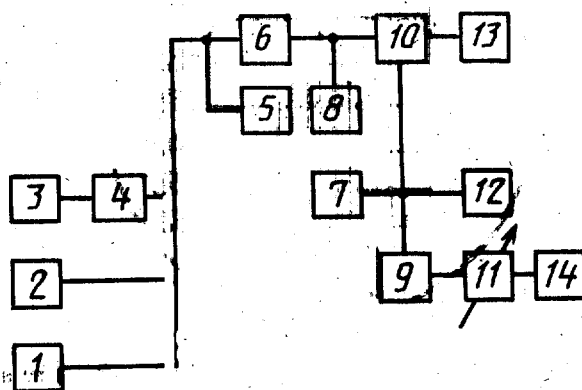
Структурная схема измерений внеполосных излучений радиопередатчиков воздушной подвижной службы
