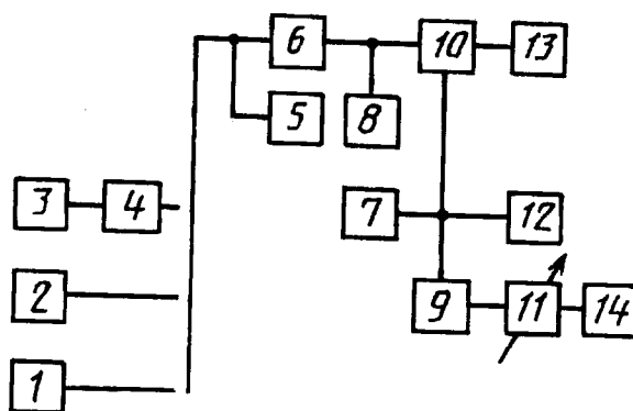
Структурная схема измерений внеполосных излучений радиопередатчиков воздушной подвижной службы
