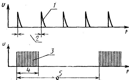
Пачки испытательных наносекундных импульсов
