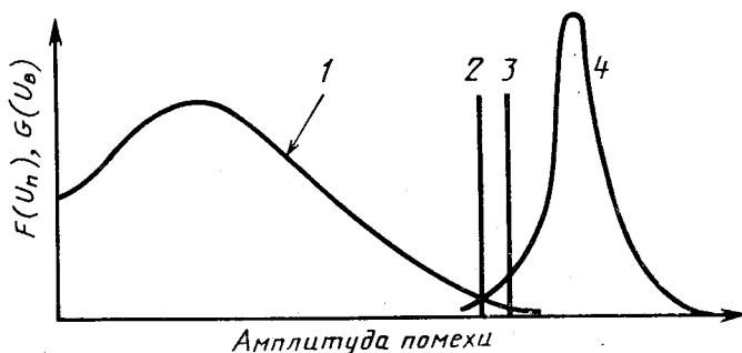
Соотношение между уровнем электромагнитных помех и уровнями помехоустойчивости, электромагнитной совмести- мости и восприимчивости ТС
