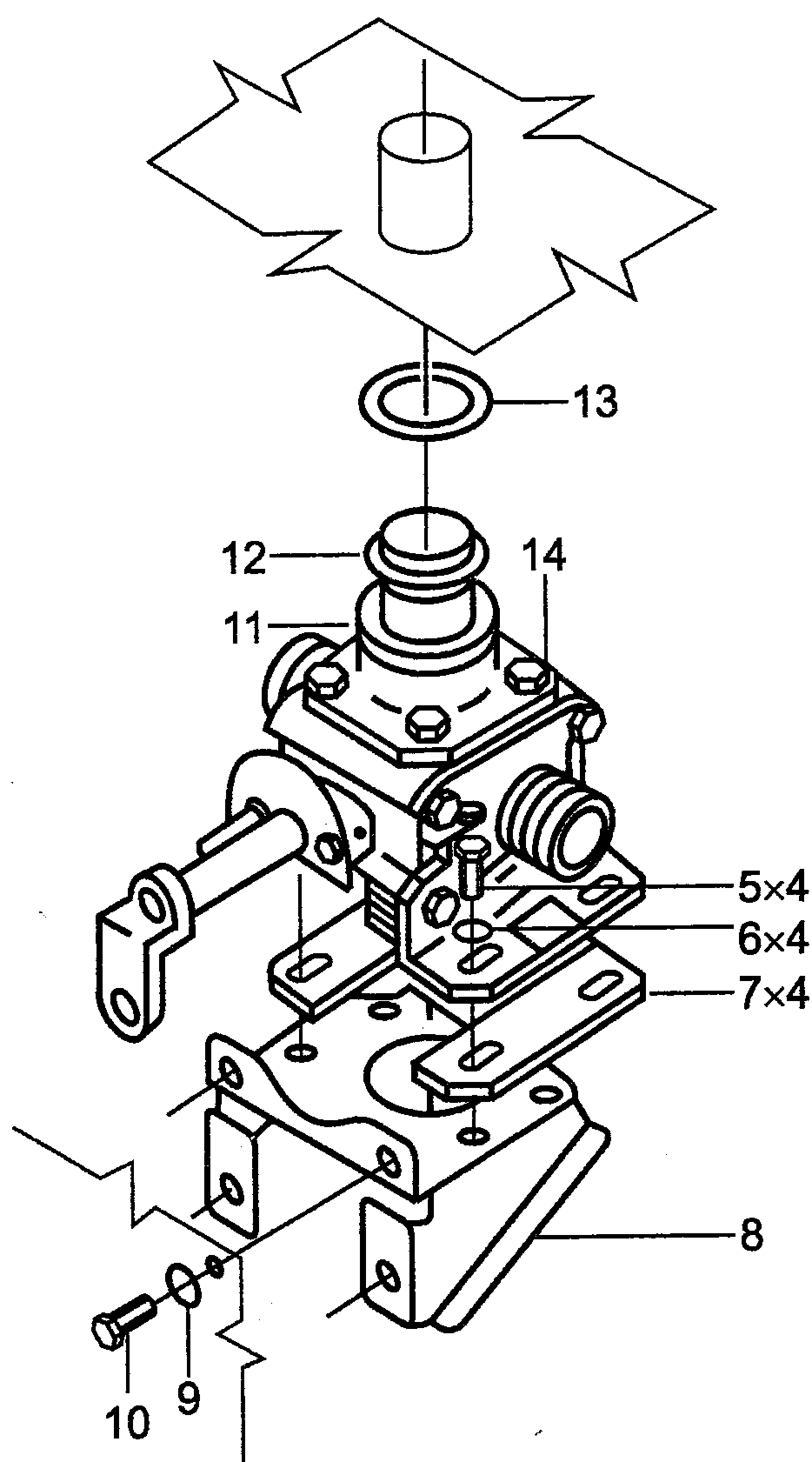
Рисунок А.1 — Пример указания количества одинаковых деталей
