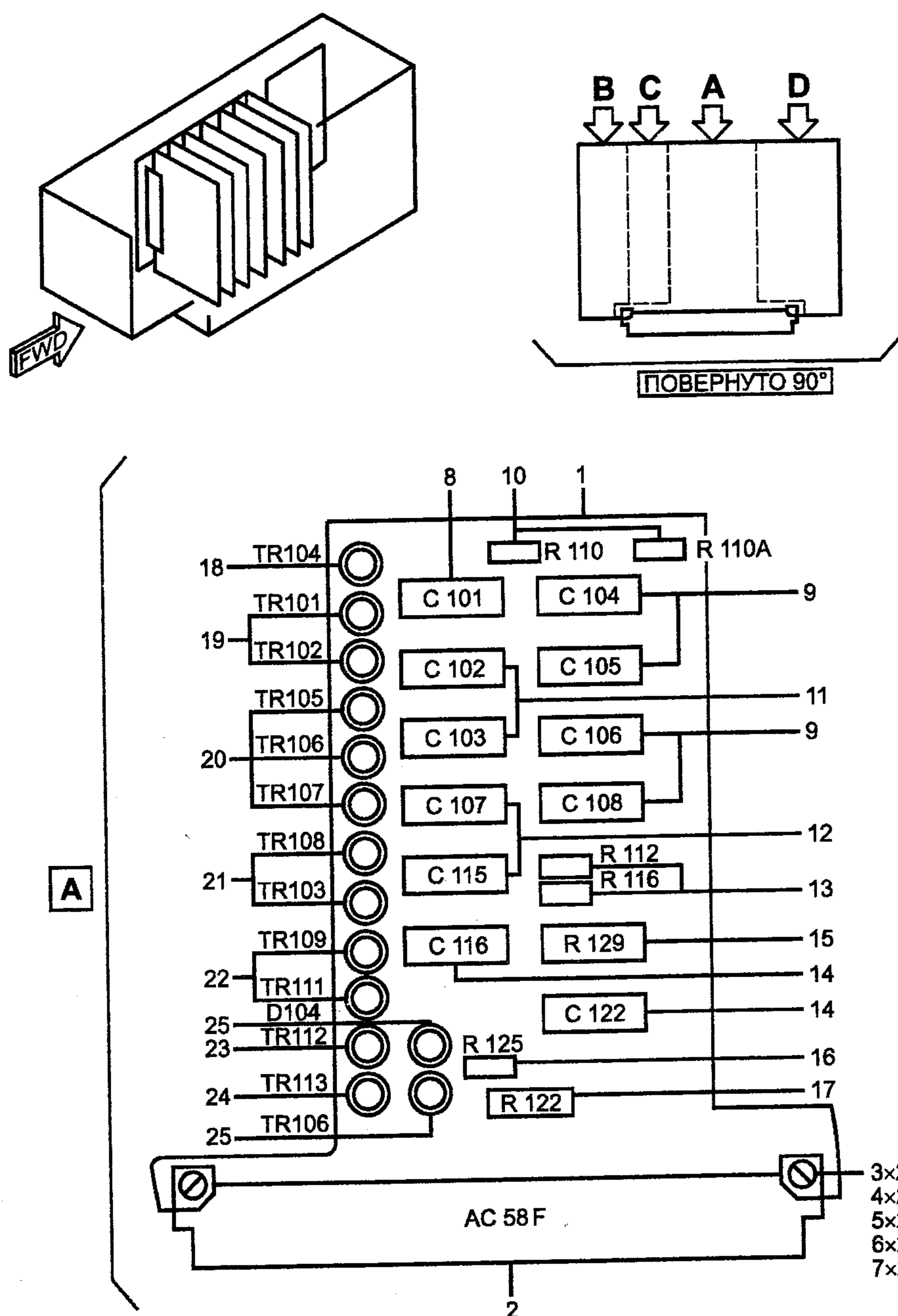
Рисунок А.3 — Пример идентификации электрических и электронных компонентов
