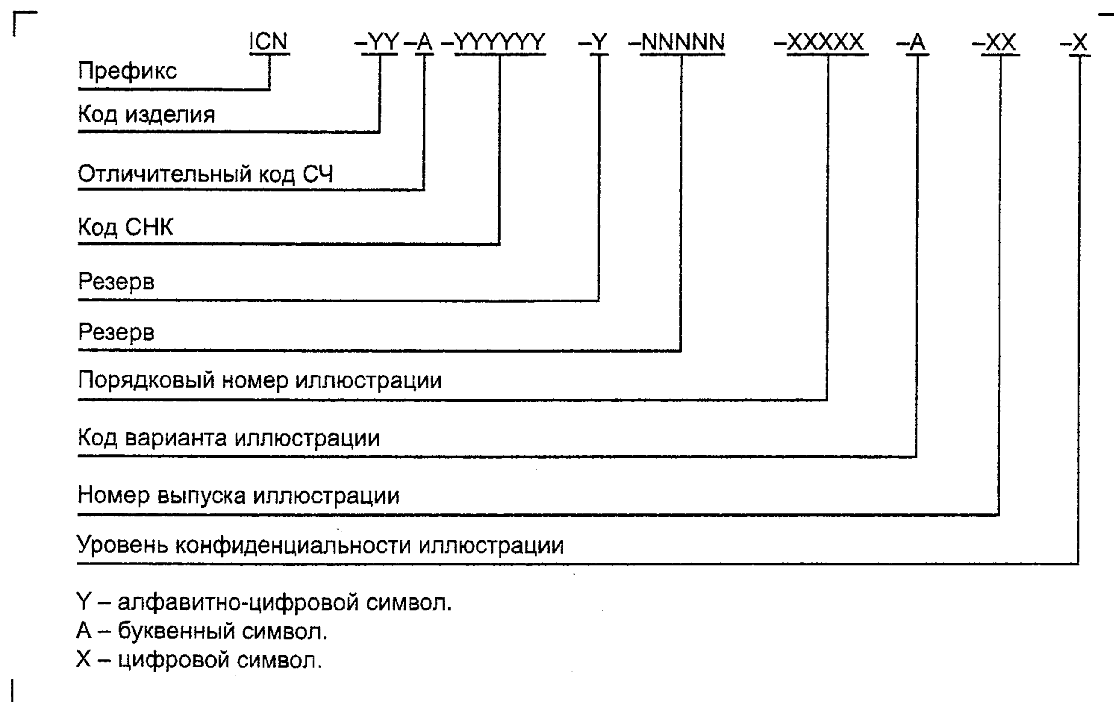
Рисунок Г.2 — Структура обозначения иллюстрации
